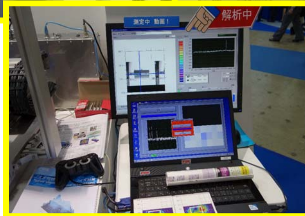
電子回路基板のノイズ放射を測定するシステム
