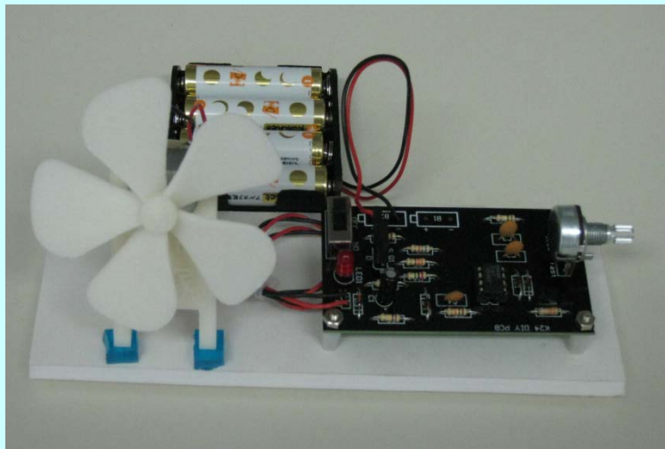
DCモータ駆動装置 完成！
